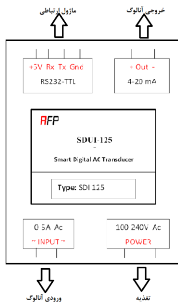
شکل ۲- نمای اتصالات دستگاه
