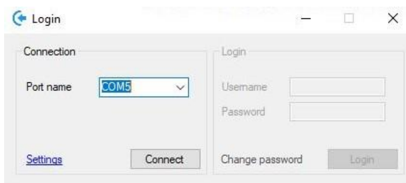
شکل ۷- پنجره LOGIN
